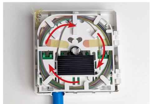
4D Fasern im Uhrzeigersinn einlegen und befestigen.
