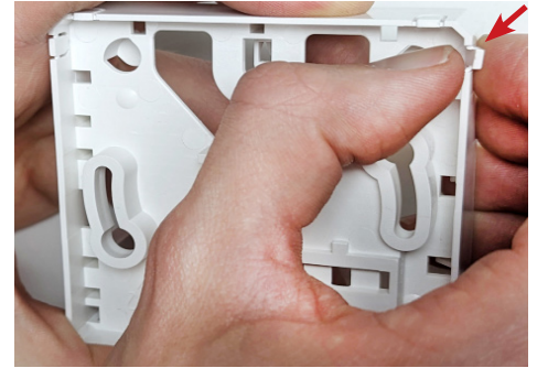
5B Eine der seitlichen Aussparungen ausbrechen.
