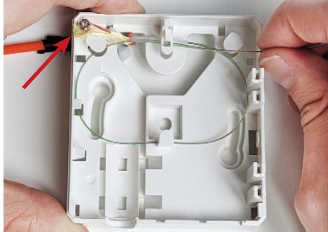
5D Fasern einmal in Halbkreis einlegen. Falls nötig Fasern befestigen. Schraube ansetzen, mit Kevlarn umwickeln. Schraube festziehen, Kevlarn kürzen (roter Pfeil).
