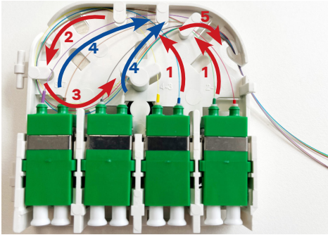
3C Fasern der zwei linken Kupplungen gemäß Abbildung einlegen (4 - 5).
