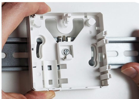
7C ARCA XS Anschlussdose auf Hutschiene aufklipsen.
