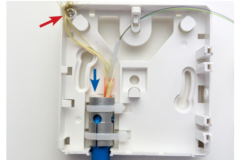
4A WGT (Gas-Wasser-Block) mit Kabelbinder am Anschlag der Ausbuchtung abfangen (blauer Pfeil). Absetzlänge des Kabels mind. 1 m. Bündel 2 cm nach WGT absetzen. Schraube ansetzen, mit Kevlarnummern umwickeln. Schraube festziehen, Kevlarnummern kürzen (roter Pfeil). Zubehör: Micro Tube Endmuffe WGT 7/4 (Art.Nr. 951272) Micro Tube Endmuffe WGT 10/6 (Art.Nr. 951273)
