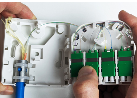
4B Tray in den Dosenboden einklippen.
