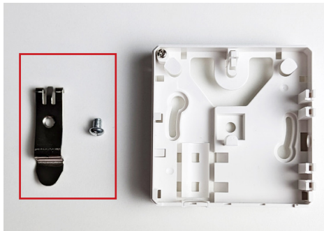
7A Zubehör: Hutschienenhalter Metall (Art.Nr. 971372)
