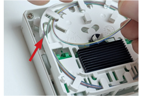
3E Fasern von Kupplungsebene auf Spleißebene des Trays führen.
