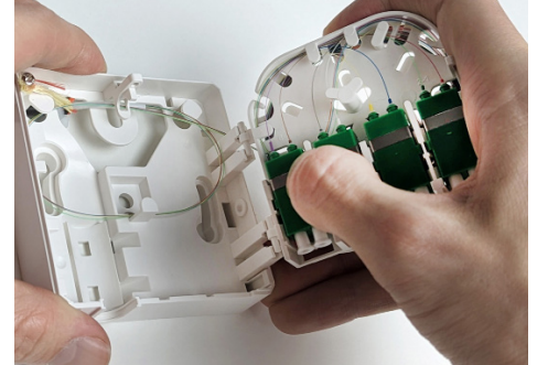
5E Tray in den Dosenboden einklippen.
