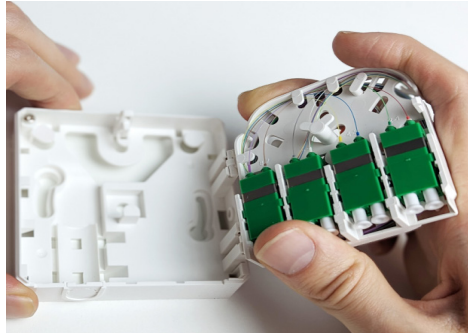
3D Tray in den Dosenboden einklippen.
