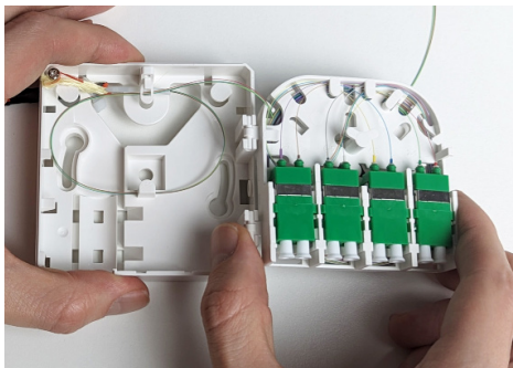
5F Fasern auf die Oberseite (Spleißebene) des Trays führen.
