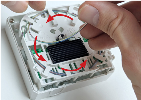
3F Fasern gegen Uhrzeigersinn einlegen.
