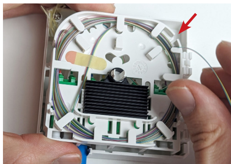
4C Fasern unter dem Niederhalter auf das Tray führen.
