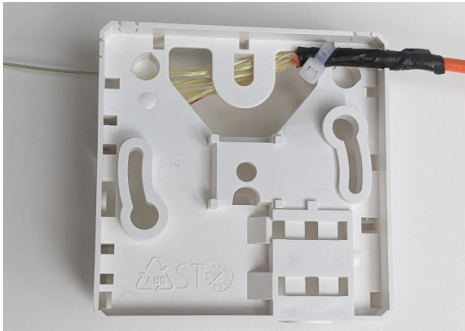
5C Kabel mit geeignetem Material ummanteln und mit Kabelbinder befestigen. Mindestens 1 m Kabel absetzen und Bündel nach 2 cm innerhalb der Anschlussdose öffnen.
