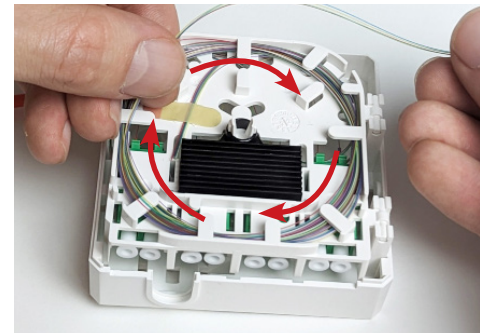
5H Fasern im Uhrzeigersinn einlegen.
