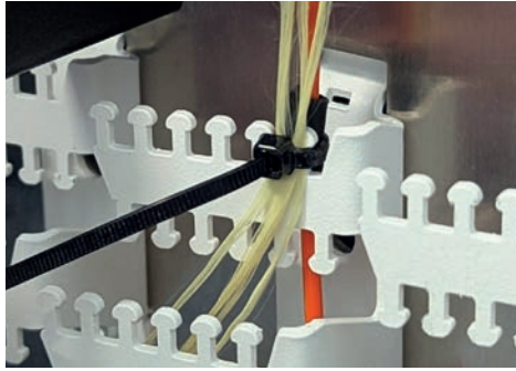
6G Kabel abisolieren und inkl. dem Aramidgarn mit Kabelbinder an Abfangung befestigen. Tipp: Beginnen Sie mit dem hintersten, innersten "T-Zapfen". Material: Kabelbinder 96/2,5 mm (Art. Nr. 970333)
