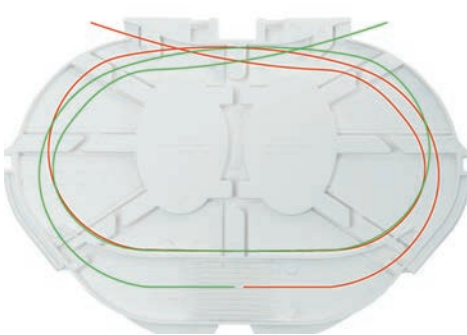
6J Faserführung in der Spleisskassette.
