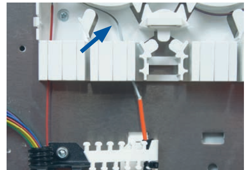
6H Kabel 10 mm unterhalb des Bündeladerhalters absetzen.
