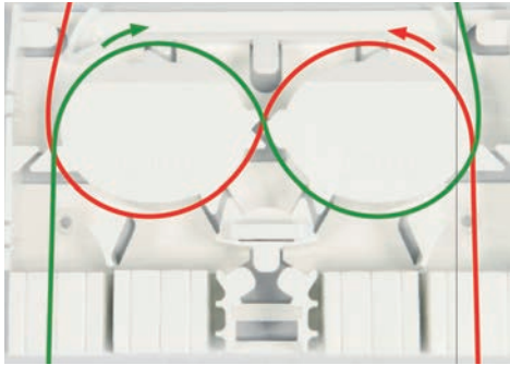
6I Beispielhafte Faserführung im Mixer. Absetzlänge der Fasern ca. 2 m
