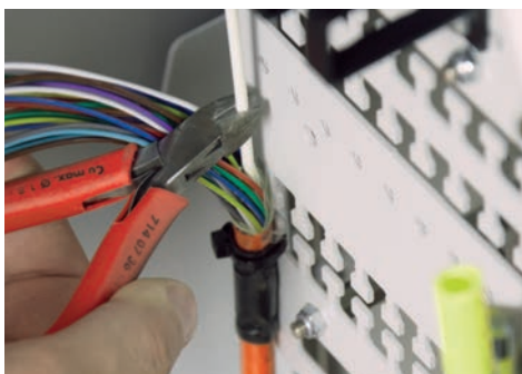
4D Zentralelement passend zur Abfangung (4E) kürzen. Werkzeug: Seitenschneider
